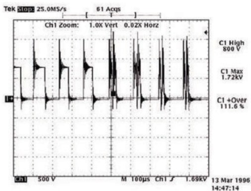
Figura 3. Fenómeno de onda reflejada presentado en la entrada del motor
